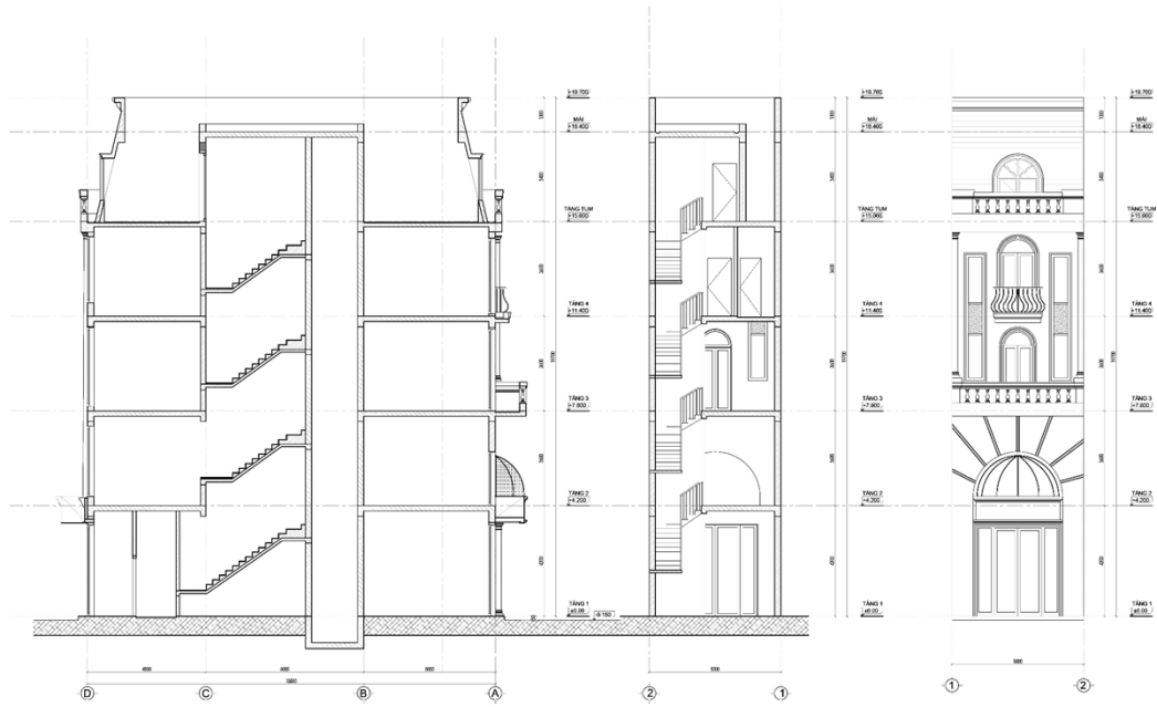
MẶT CẮT - MẶT ĐỨNG KIẾN TRÚC
