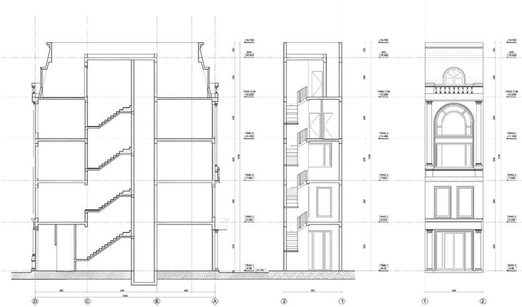
MẶT CẮT - MẶT ĐỨNG KIẾN TRÚC
