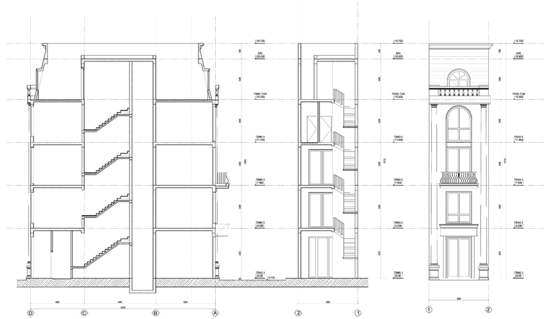
M Ặ T C Ắ T - M Ặ T Đ Ứ N G K I Ế N T R Ứ C
